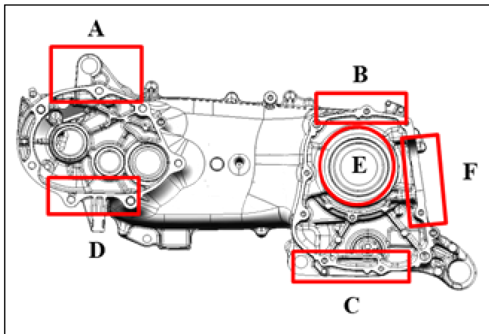
Gambar 4 Titik Bagian Pengukuran Ketebalan Dinding Part
